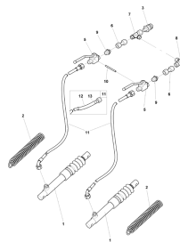
ETB-010421, Hydrauliczna regulacja zasuw I
