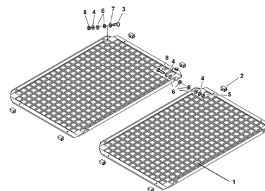
ETB-010438, Krata ochronna
