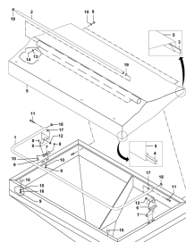
ETB-010436, Składana plandeka
