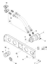
ETB-010433, Napęd hydr.
