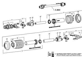
ETB-0000005675, Wałek przegubowo-teleskopowy EJ684 -W 100 E 710 mm, 1 3/8 cala, 6 sztuk
