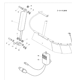
ETB-010426, Elektryczna regulacja szerokości rozsiewu od 11.2010
