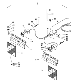
ETB-010439, Oświetlenie tylne
