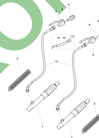
ETB-010422, Hydrauliczne sterowanie kombinowane I
