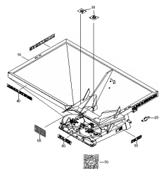
ETB-010416, Rama ze zbiornikiem
