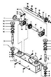
ETB-010432, Przekładnia / II
