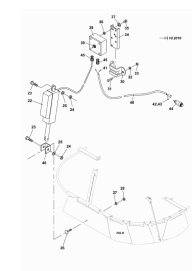
ETB-010427, Elektryczna regulacja szerokości rozsiewu do 10.2010
