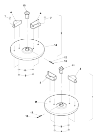
ETB-010429, Tarcze rozsiewające
