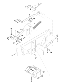
ETB-010419, Dźwignia nastawcza i zsypy z prawej strony
