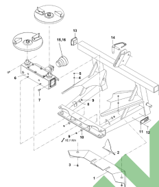
ETB-010418, Osłona blaszana
