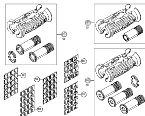
ETB-010428, Uchwyt węży hydraulicznego
