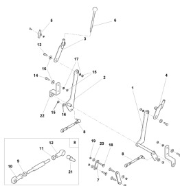
ETB-010424, Sterowanie ręczne
