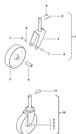
ETB-010441, Urządzenie transportowe
