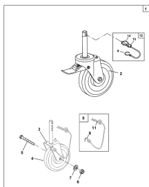
ETB-010440, Kółka transportowe do ZA, hamowane od 05.2006!
