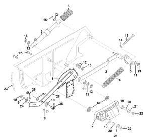
ETB-010420, Dźwignia nastawcza i zsypy z lewej strony
